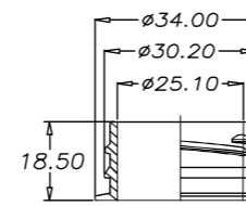
30/25 - 3-Start
